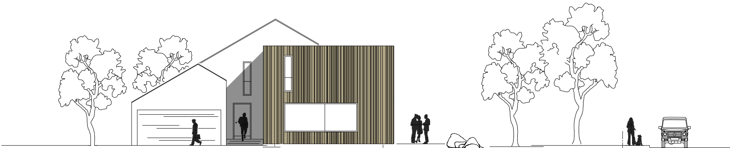
Ansicht WEST 1_150
